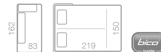
DIMENSIONS DU CENTO-60
